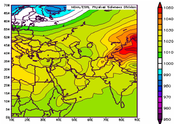
شکل (۳) نقشه‌های روز ۳، ۴ و ۵ ژانویه ۲۰۰۷ (افقی) در سه تراز سطح زمین، ۸۵۰ هکتوپاسکال و ۷۰۰ هکتوپاسکال (عمودی)
