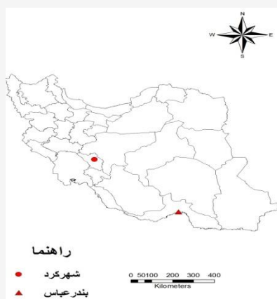
شکل (۱) موقعیت ایستگاه‌های بندرعباس و شهرکرد در ایران
