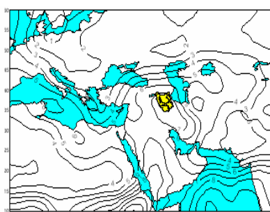
شکل (۶) نم ویژه تراز ۸۵۰ هکتوپاسکال ساعت ۰۰۰۰ گرینویچ ۲۰۰۳/۱۱/۱۱
