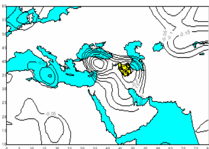
شکل (۷) میدان حرکات بالاسو تراز ۵۰۰ H ساعت ۰۰۰۰ گرینویچ ۲۰۰۳/۱۱/۱۱
