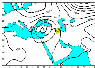
شکل (۳) نقشه سطح ۸۵۰ H ساعت ۰۰۰۰ گرینویچ ۲۰۰۳/۱۱/۱۱
