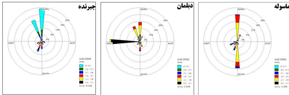
شکل (۲) گل‌بادهای سالانه ایستگاه‌های همید ماسوله، چیرنده و دیلمان (تهیه نگارندگان).
