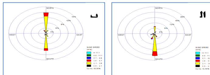
شکل (۱۰) تفاوت در رفتار باد فراشیب و فروشیب تحت تاثیر تغییر فصل. الف. گل باد ساعت ۱۵ UTC در ماه آبان و ب. گل باد ساعت ۱۵ ماه شهریور.
