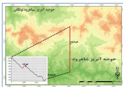
شکل (۵) نقشه و نیمرخ توپوگرافی جیرنده (تهیه نگارندگان).
