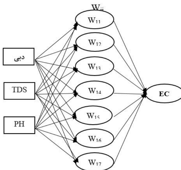
شکل ۴- نقشه شماتیک الگوریتم انتخابی ANN
