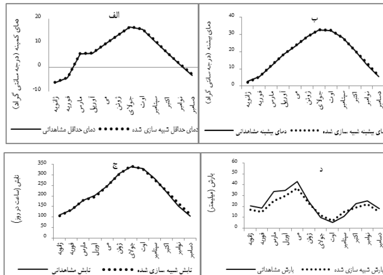
شکل ۲- مقایسه مقادیر نتایج حاصل از مدل و دیده بانی شده برای دماهای کمینه (الف)، بیشینه (ب)، تابش (ج) و بارش (د) در حوضه آبریز تسوج (۲۰۱۲-۱۹۸۴)
