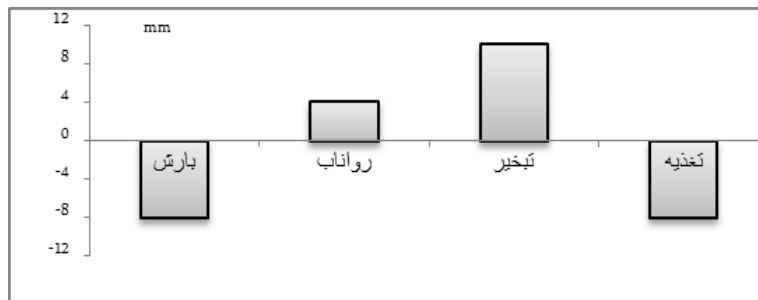
شکل ۵- اختلاف میانگین سالانه بارش، رواناب، تأخیر و تغذیه برای دوره ۲۰۲۲-۲۰۱۳ نسبت به دوره مبنا در حوضه آبریز تسوج با استفاده از مدل HADCM۳ و سناریوی A۲
