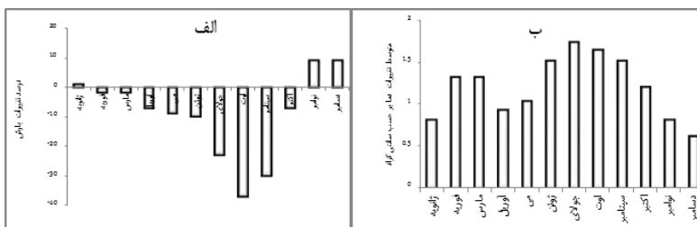
شکل ۴- تغییرات پیش بینی شده برای بارش (الف) و دما (ب) برای دوره ۲۰۱۳-۲۰۳۰ نسبت به دوره مینا در حوضه آبریز تسوج با استفاده از مدل HADCM۳ و سناریوی A۲
