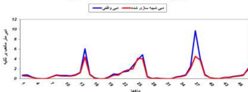
نمودار دبی واقعی و شبیه‌سازی شده در دوره اعتبارسنجی
