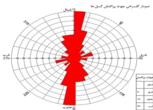
شکل ۲. دیاگرام گلسرخی خطواره‌های گسلی محدوده مورد مطالعه
