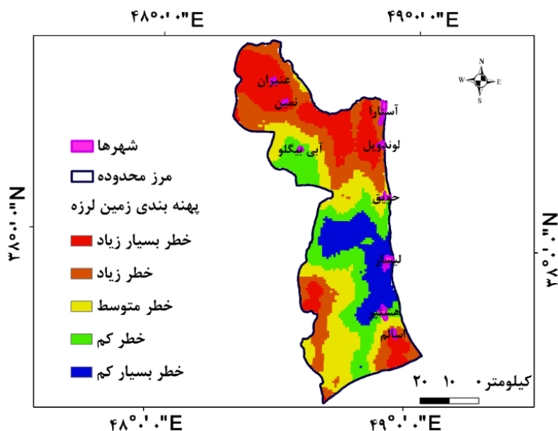
شکل ۱۳. نقشه پهنه‌بندی خطر زمین لرزه در منطقه مورد مطالعه
