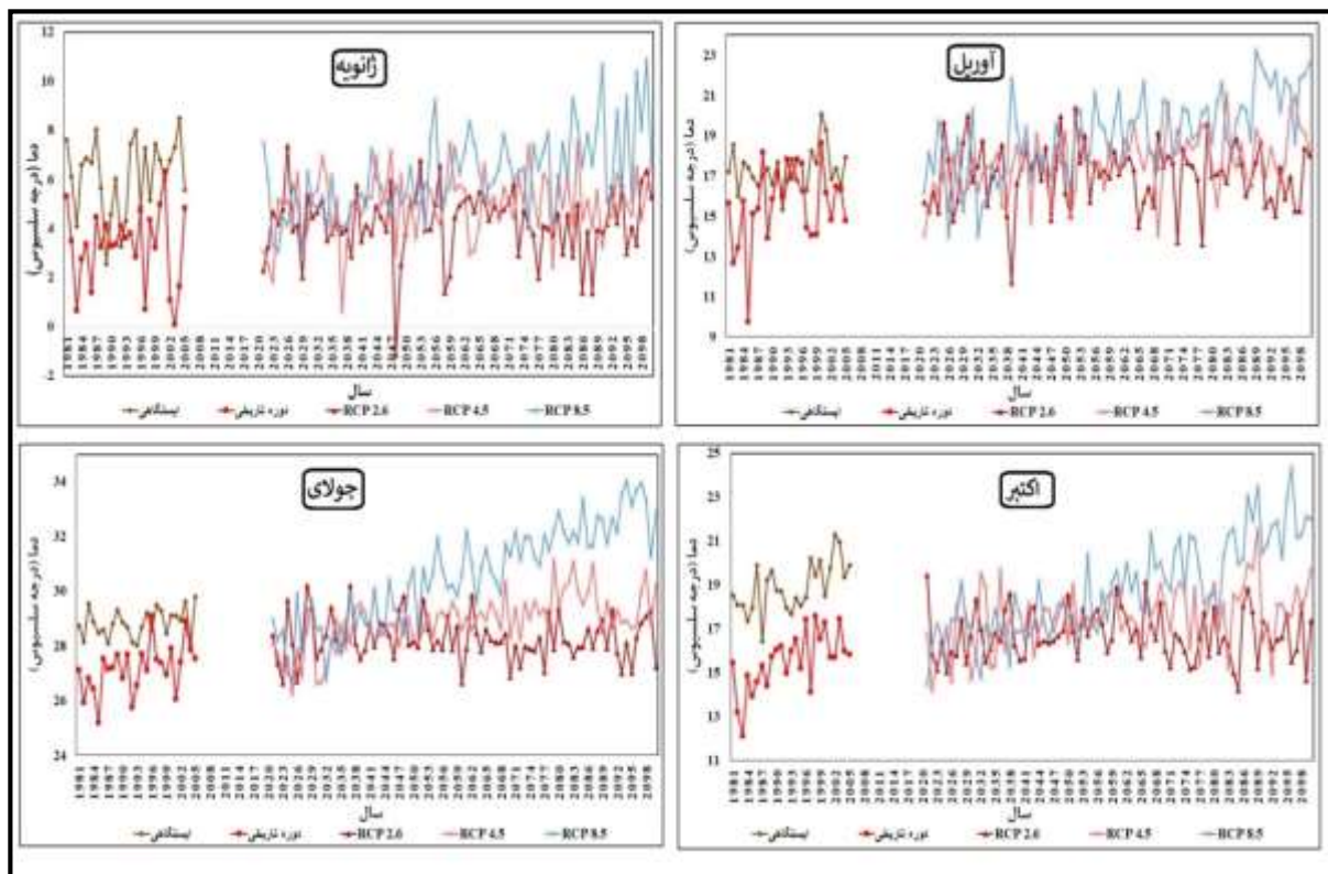
شکل (۳): شیب روند دمای هوا طی دوره مشاهداتی (۱۹۸۰-۲۰۰۵) و آینده (۲۰۲۱-۲۱۰۰) براساس داده‌های ایستگاهی و داده‌های مدل MPI-ESM-LR تحت سناریوهای واداشت تابشی RCPs (به دلیل بالا بودن تعداد نمودارها، اولین ماه هر فصل را به عنوان نمونه ارائه
