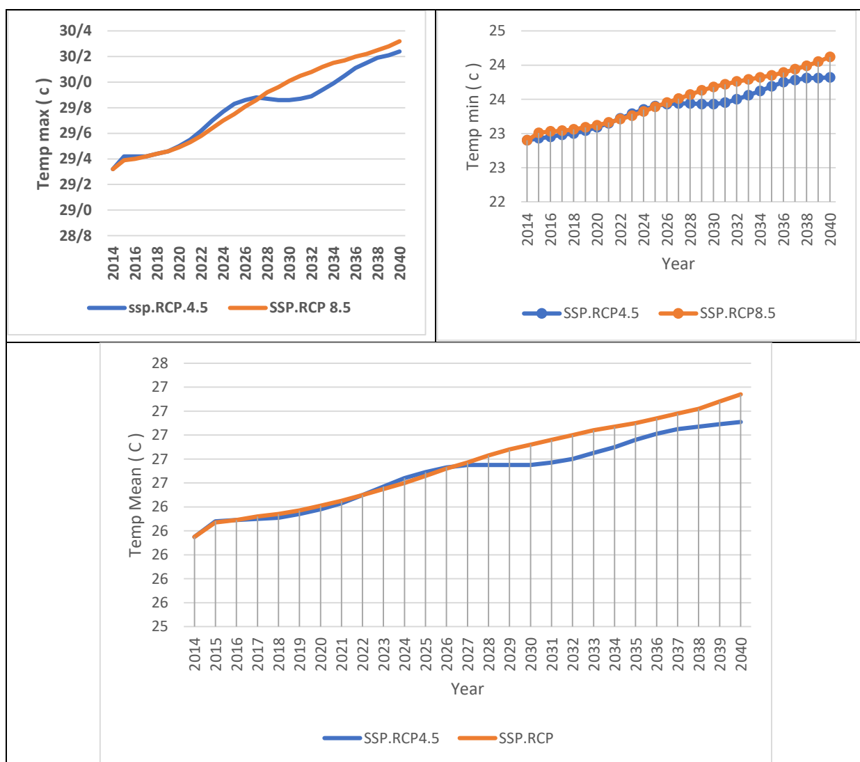
شکل(۶) نمودار تغییرات دمای کمینه، میانگین و بیشینه استان بوشهر در سناریوهای ۴,۵ و ۸,۵ (۲۰۱۴-۲۰۴۰)
