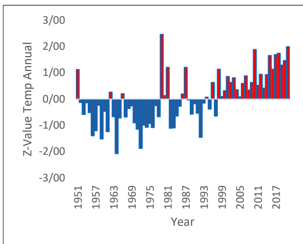
شکل ۲. آنومالی میانگین دمای سالانه ایستگاه بوشهر
