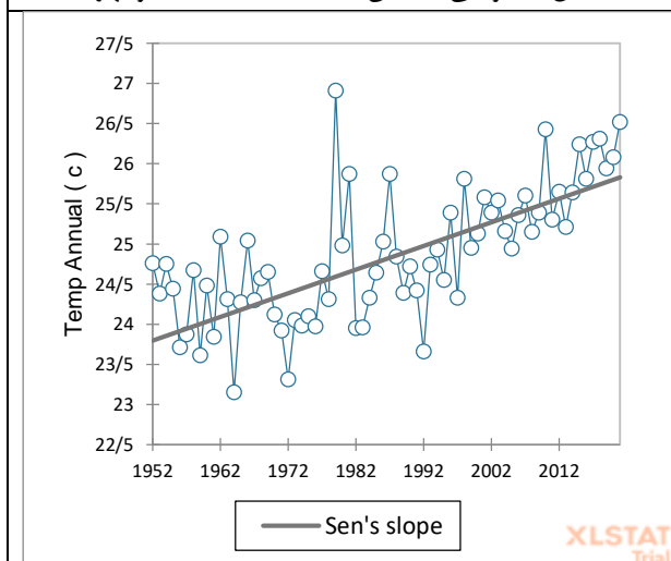
شکل ۴. سنز-شیب دمای سالانه ایستگاه بوشهر
