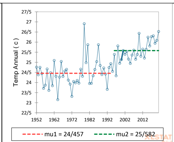
شکل ۳. آزمون Pettitt دمای سالانه ایستگاه بوشهر
