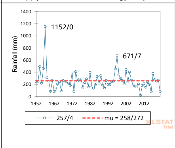
شکل ۵. آزمون Pettitt بارش سالانه ایستگاه بوشهر
