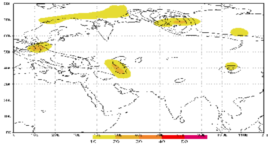
شکل (۷) نقشه رودیاد سطح ۲۵۰ هکتوپاسکال در ساعت ۰۰:۰۰
