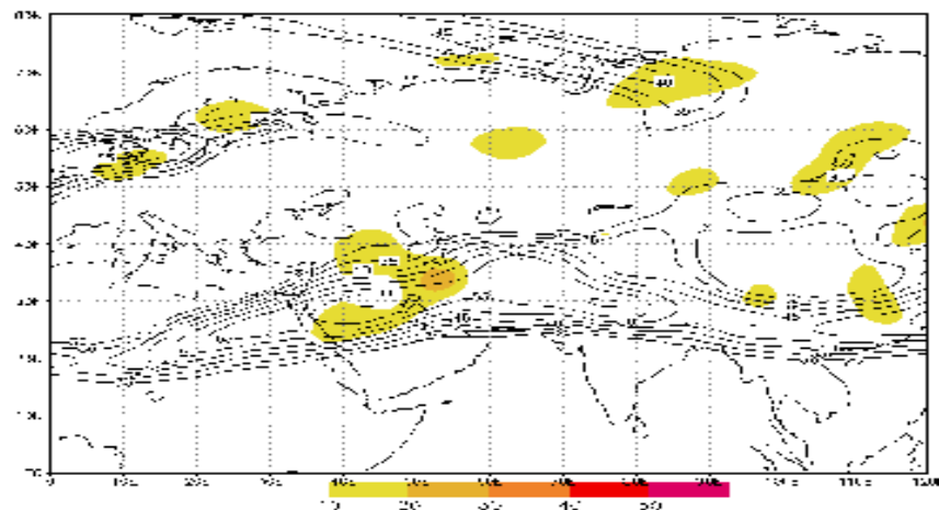
شکل (۸) نقش رودیاد سطح ۳۰۰ هکتوپاسکال در ساعت ۱۸:۰۰
