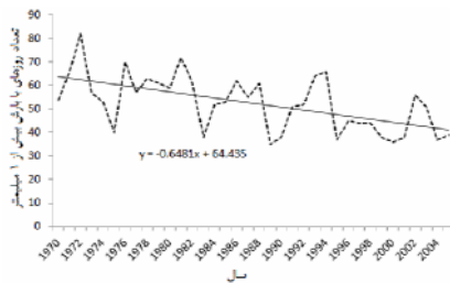
شکل (۱۰) روند تغییرات تعداد روزهای با بارش بیش از ۵ mm در ایستگاه تبریز در دوره آماری ۱۹۷۰-۲۰۰۵ از شکل (۱۱) روند تغییرات تعداد روزهای با بارش بیش از ۱ mm در ایستگاه تبریز در دوره آماری ۱۹۷۰-۲۰۰۵
