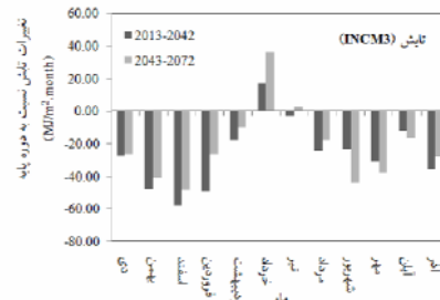
شکل (۲) پیش‌بینی تغییرات ماهانه پارامترهای هواشناسی تحت سناریوی AIB برای دو دوره ۲۰۱۳-۲۰۴۲ و ۲۰۴۳-۲۰۷۲ نسبت به دوره پایه، توسط مدل انتخابی برای هر پارامتر
