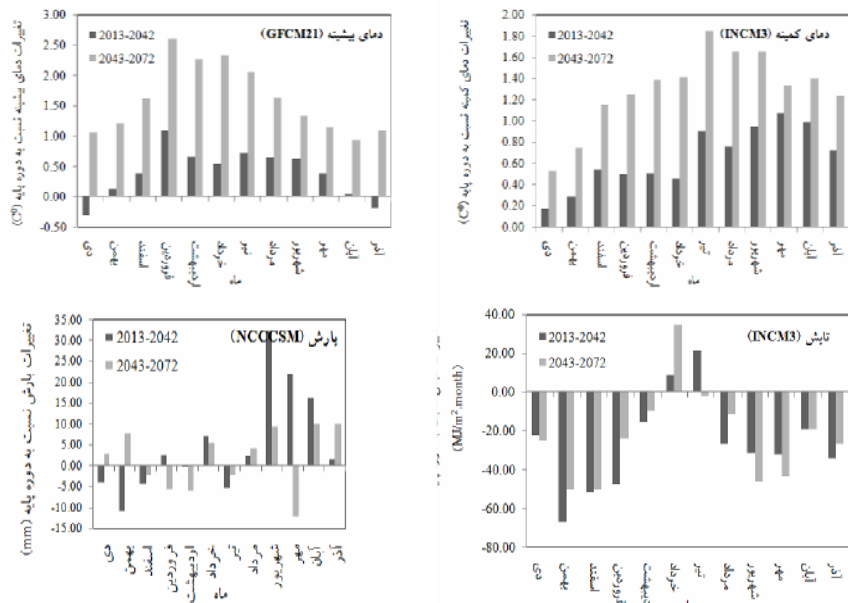
شکل (۳) پیش‌بینی تغییرات ماهانه پارامترهای هواشناسی تحت سناریوی A2 برای دو دوره ۲۰۱۳-۲۰۴۲ و ۲۰۴۳-۲۰۷۲ نسبت به دوره پایه، توسط مدل انتخابی برای هر پارامتر
