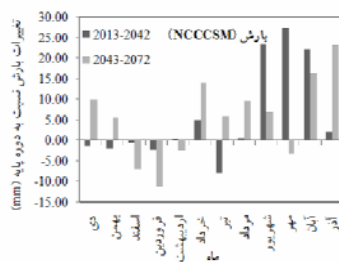
شکل (۲) پیش‌بینی تغییرات ماهانه پارامترهای هواشناسی تحت سناریوی AIB برای دو دوره ۲۰۱۳-۲۰۴۲ و ۲۰۴۳-۲۰۷۲ نسبت به دوره پایه، توسط مدل انتخابی برای هر پارامتر
