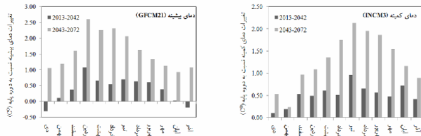
شکل (۳) پیش‌بینی تغییرات ماهانه پارامترهای هواشناسی تحت سناریوی A2 برای دو دوره ۲۰۱۳-۲۰۴۲ و ۲۰۴۳-۲۰۷۲ نسبت به دوره پایه، توسط مدل انتخابی برای هر پارامتر
