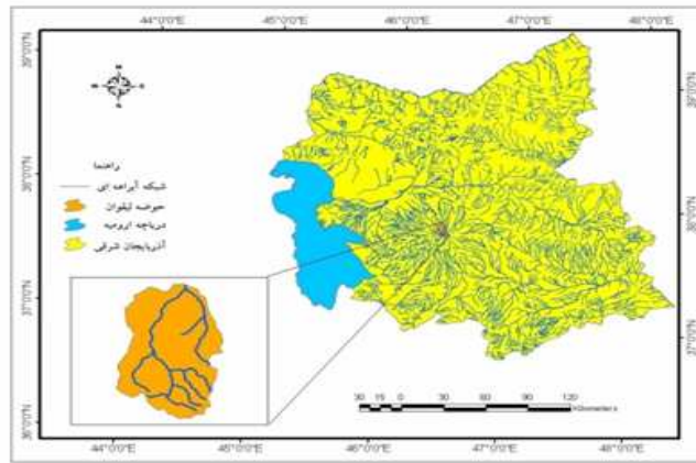
شکل (۲) موقعیت جغرافیایی منطقه مورد مطالعه (حوضه آبریز ليقوان)
