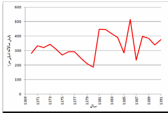
شکل (۳) بارندگی سالانه ایستگاه ليقوان در دوره آماری ۱۳۶۹-۱۳۹۱
