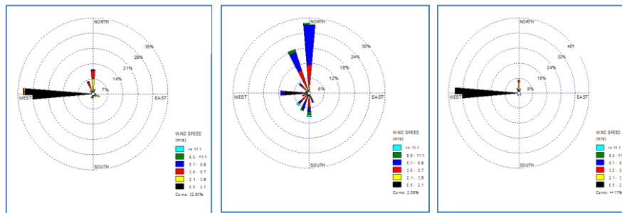
شکل (۶) سازوکار باد در امتداد دره در ایستگاه دیلمان در ساعت‌های ۰۳، ۰۹ و ۱۵ UTC نشان داده شده است. با توجه به سازوکار باد در امتداد دره، این باد در ایستگاه دیلمان، در دو ساعت ابتدایی و انتهایی روز غالب است.
